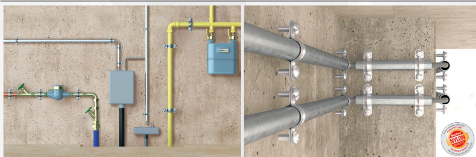
Collare per tubi CPT completo di vite e tassello SX Plus.
