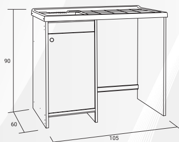
105x60 Sx Vasca bordo basso
