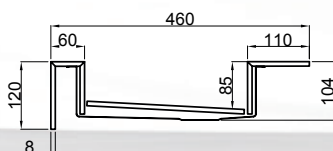
Sezione Laterale
